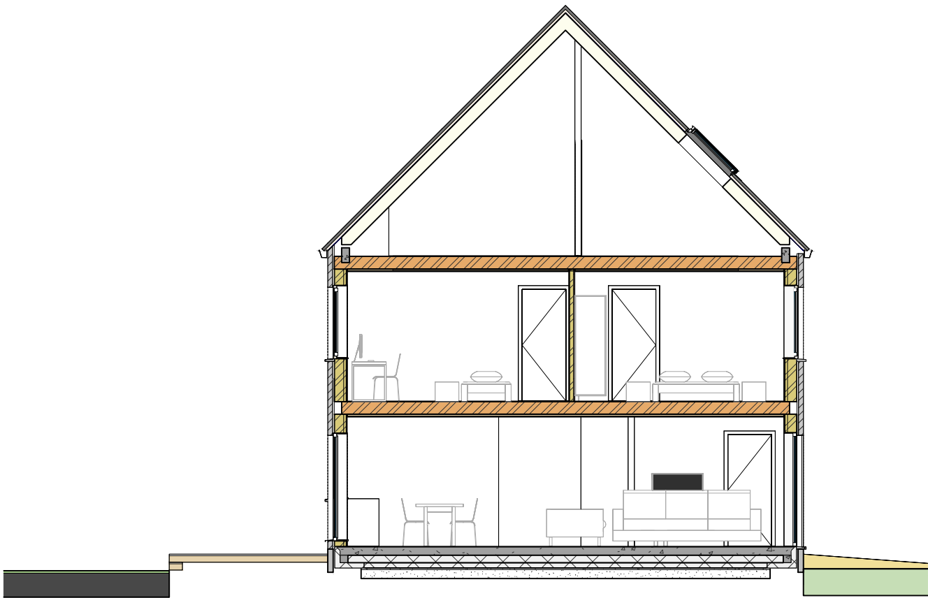
Snede Schaal 1 : 100
