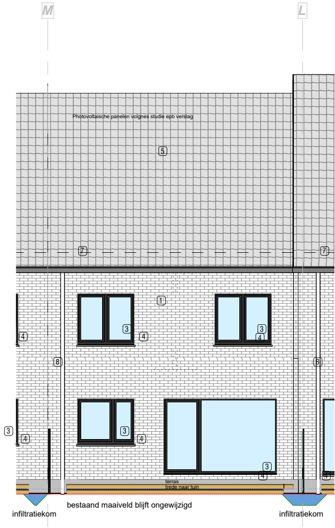
Achtergevel Schaal 1 : 100
